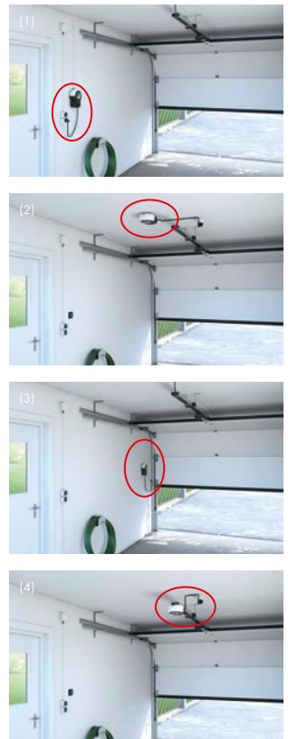
De pro + -besturing kan achter (1), aan het plafond (2), vóór (3) of direct op de looprail (4) worden gemonteerd.
